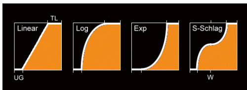
Abbildung 4.73 Transformationsfunktionen mit verschiedenen Charakteristiken.
